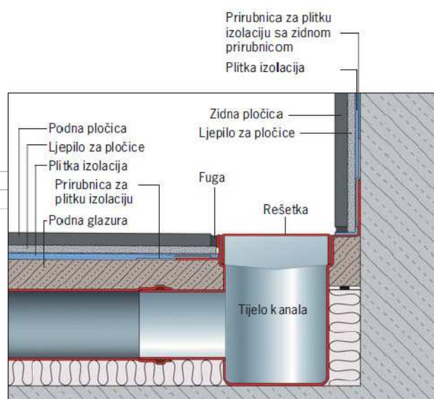
Plitka varijanta sa prirubnicom za plitku hidroizolaciju
