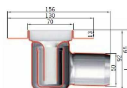
Standardna varijanta sa prirubnicom za plitku hidroizolaciju
