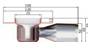
Plitka varijanta sa prirubnicom za plitku hidroizolaciju
