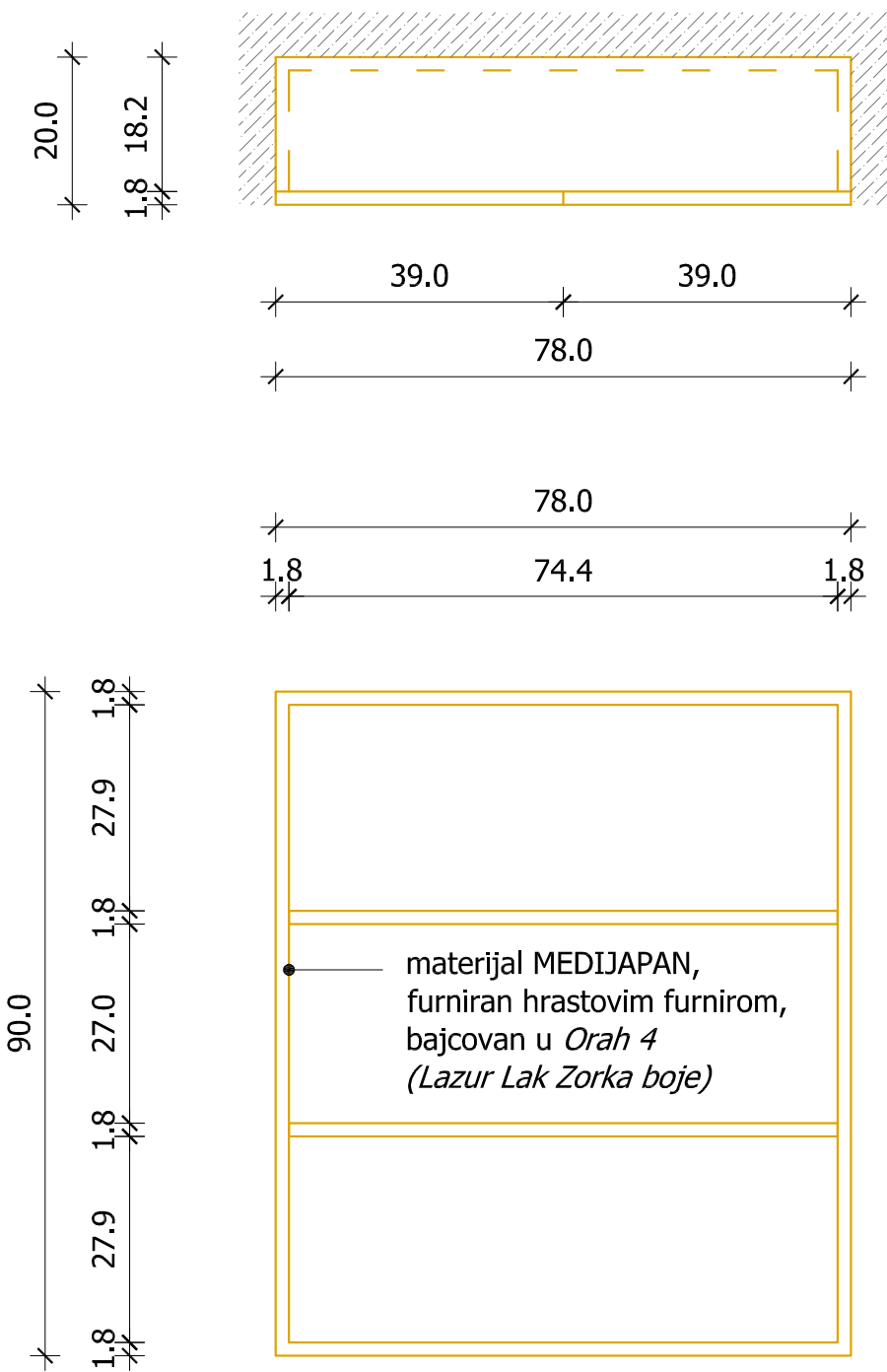
Pogled odozgo
