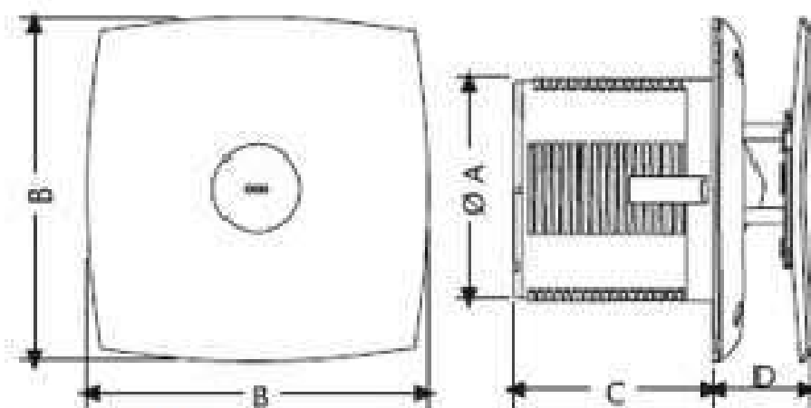
DIMENSIONES mm
