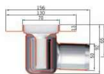
Standardna varijanta za priključkom za plitku hidroizolaciju
