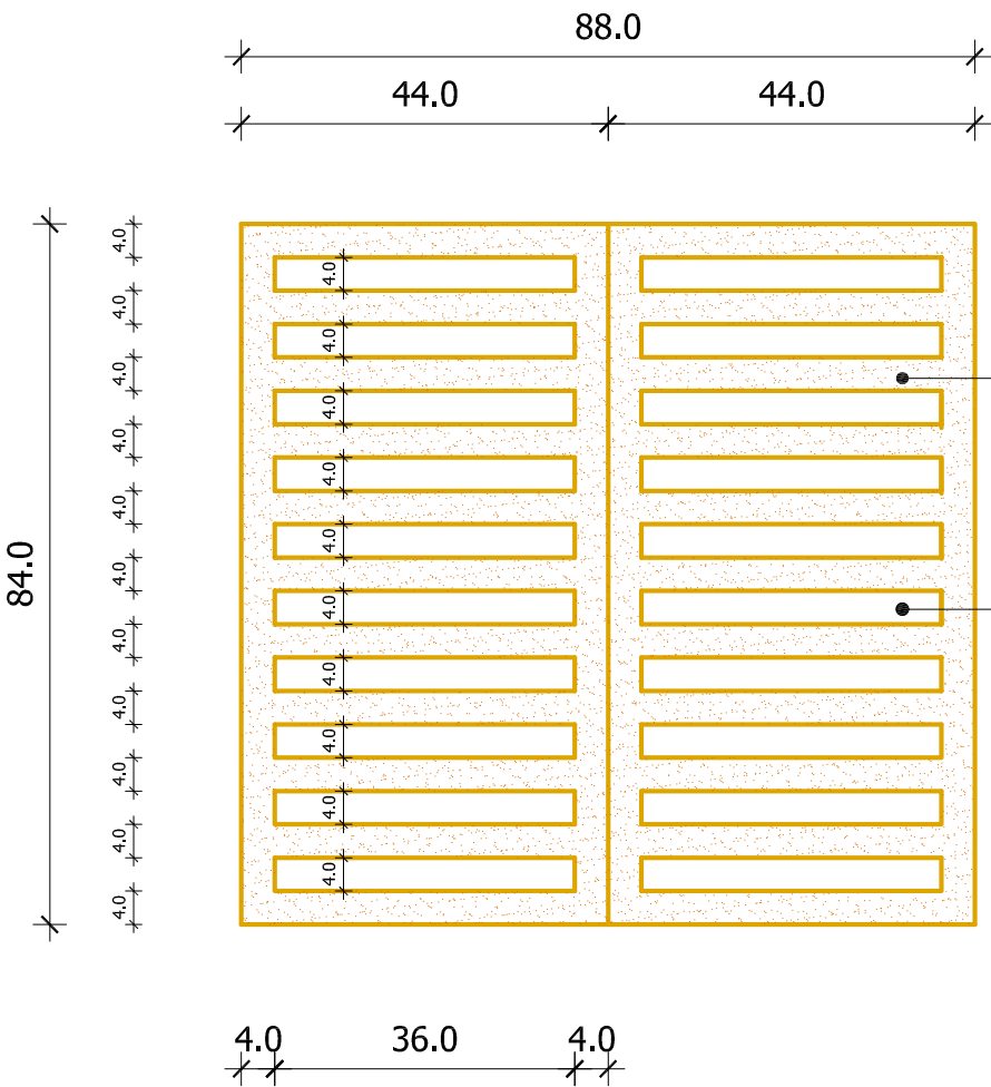
Izgled fronta
