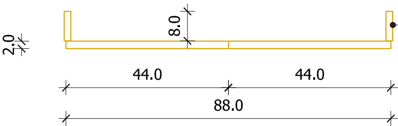
Pogled odozgo
