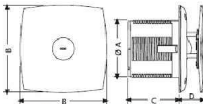
DIMENSIONES mm
