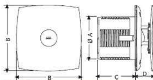
DIMENSIONES mm
