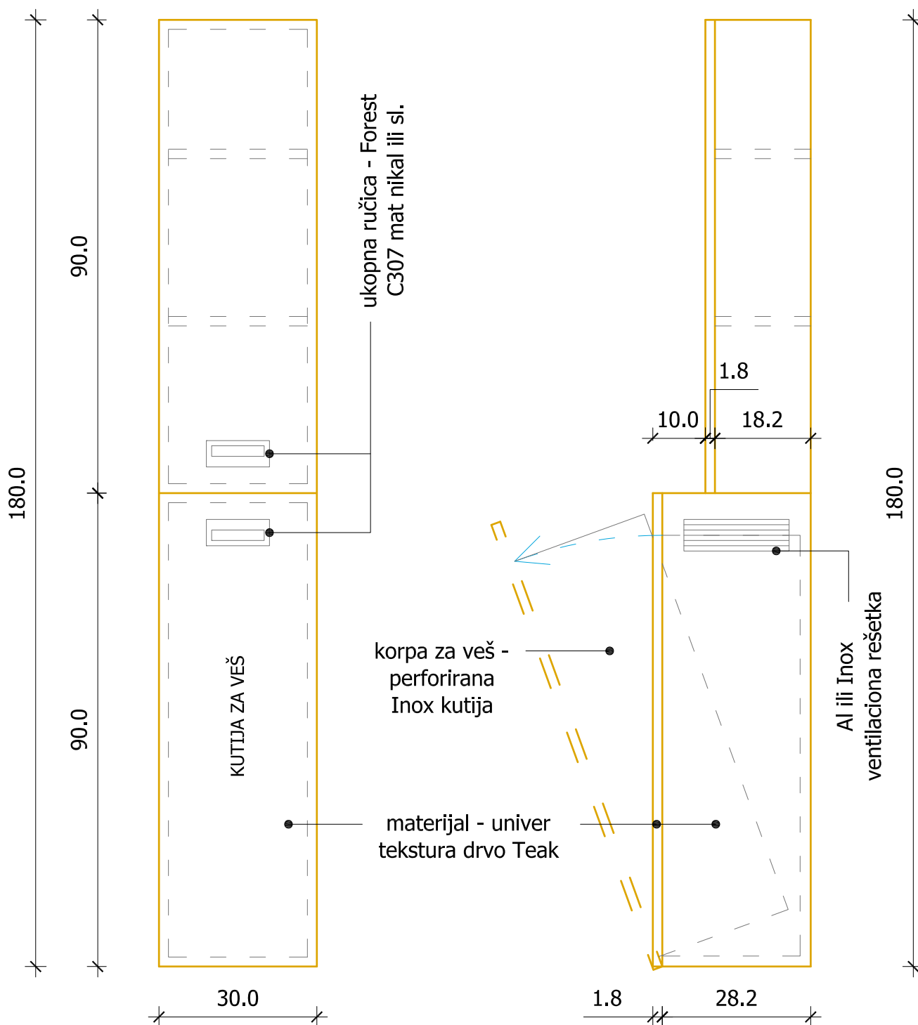
Izgled fronta
