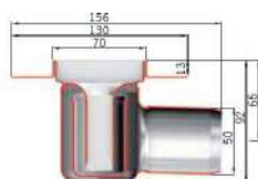
Standardna varijanta sa prirubnicom za plitku hidroizolaciju
