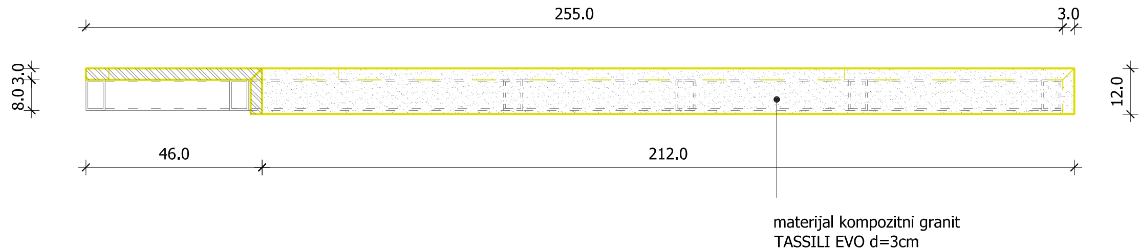
Pogled sa strane
