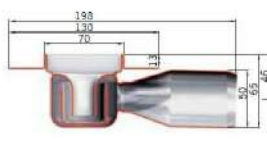
Plitka varijanta sa prirubnicom za plitku hidroizolaciju
