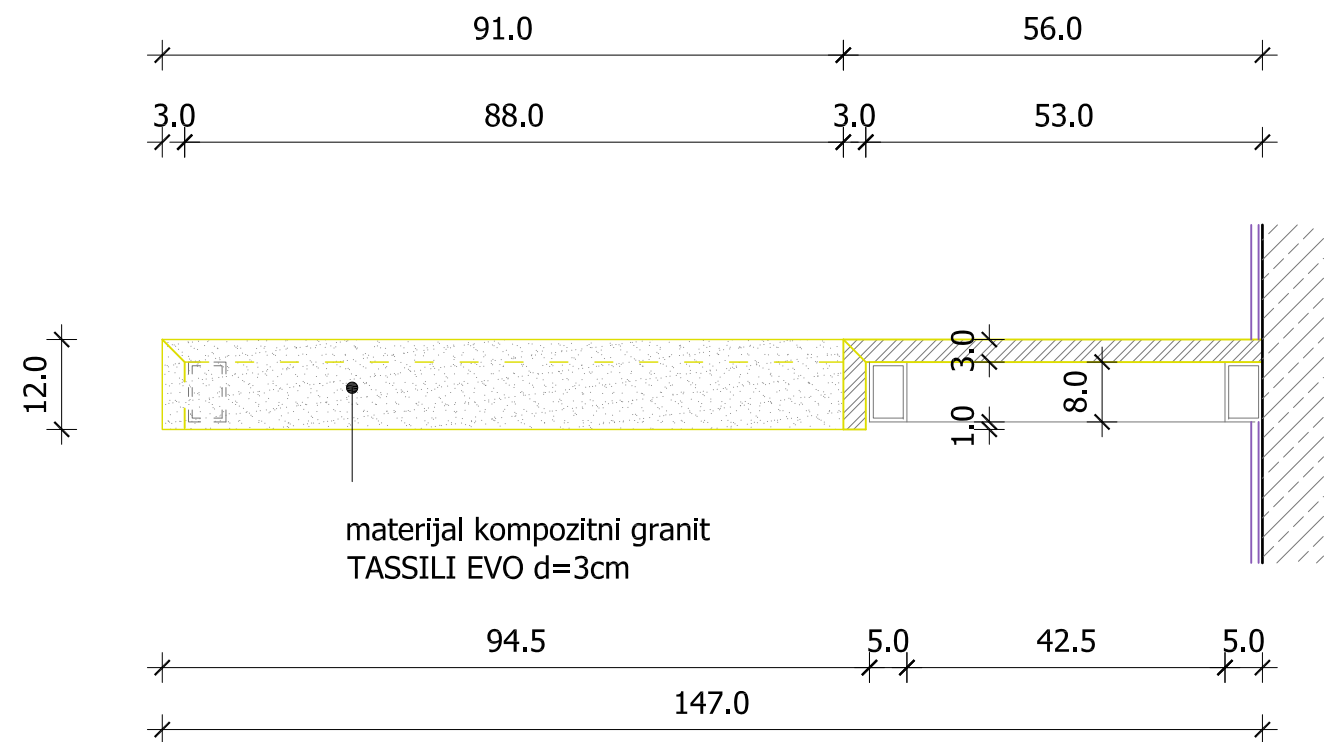
Pogled sa strane
