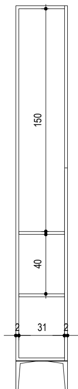
Poprečni presek
