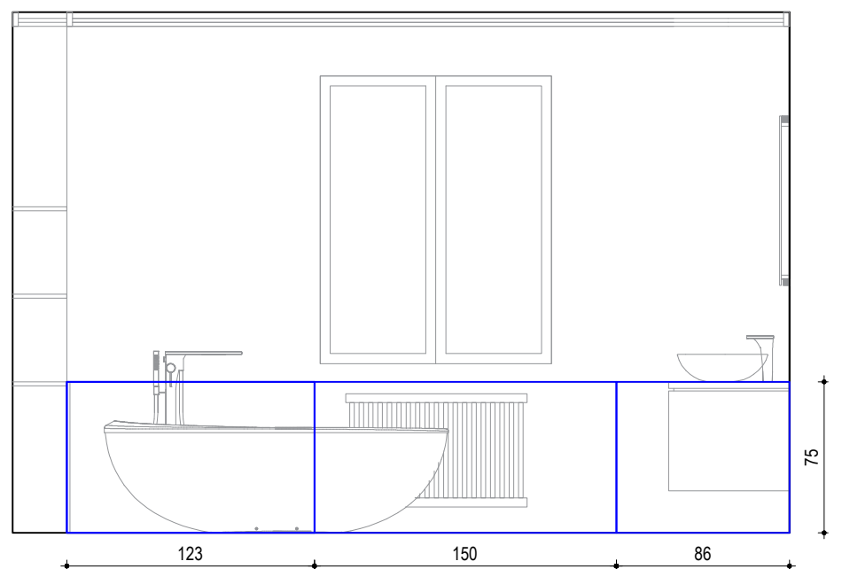
Izgled D
