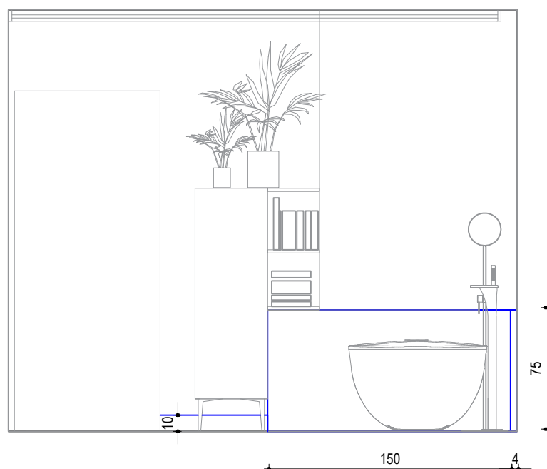
Izgled C
