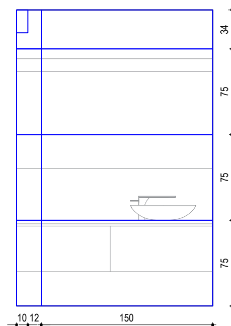
Izgled D
