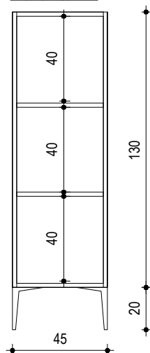
Poprečni presek
