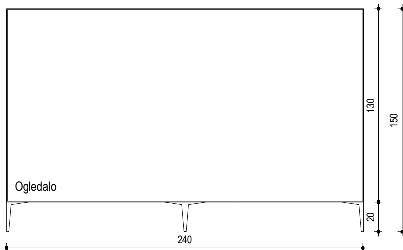
Prednji izgled
