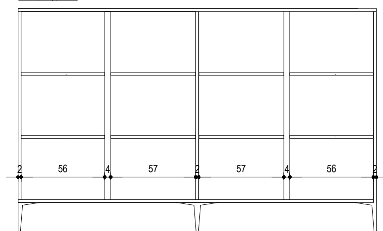
Podužni presek
