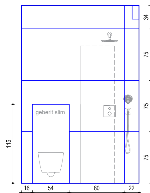
Izgled B
