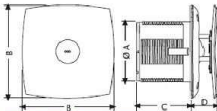
DIMENSIONES mm
